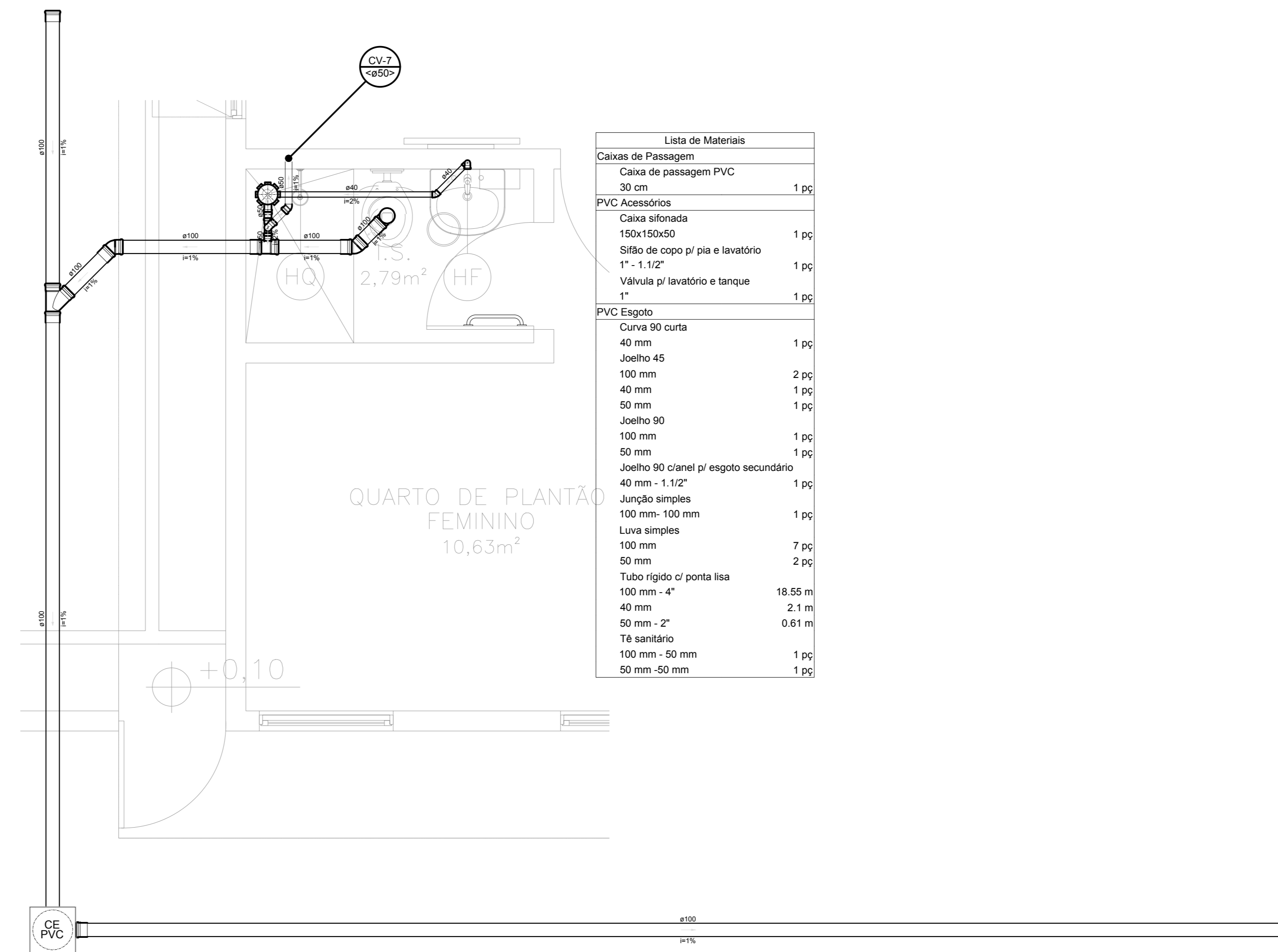
4 DETALHE S04 ESCALA 1:25
