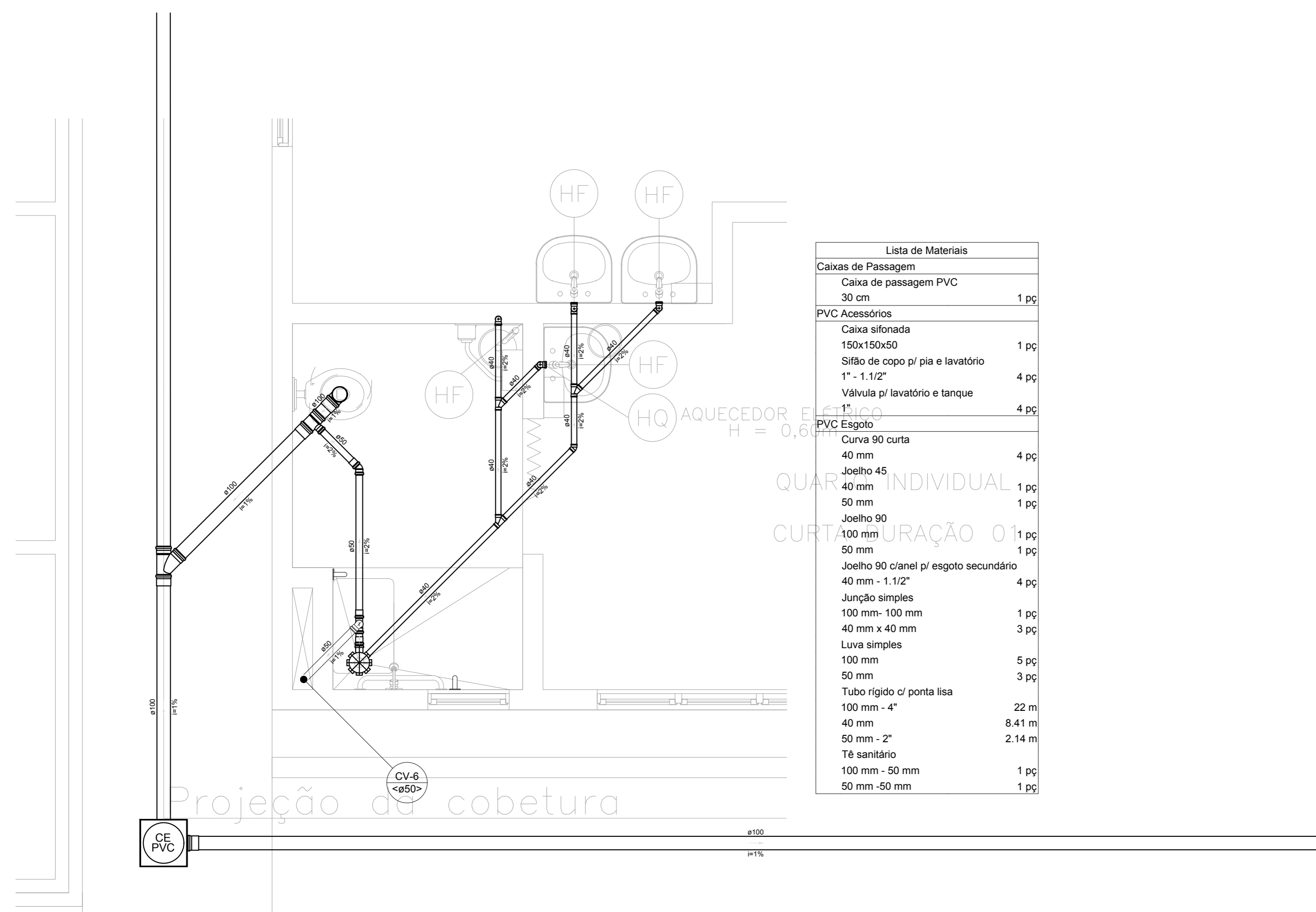
1 DETALHE S03 ESCALA 1:25
